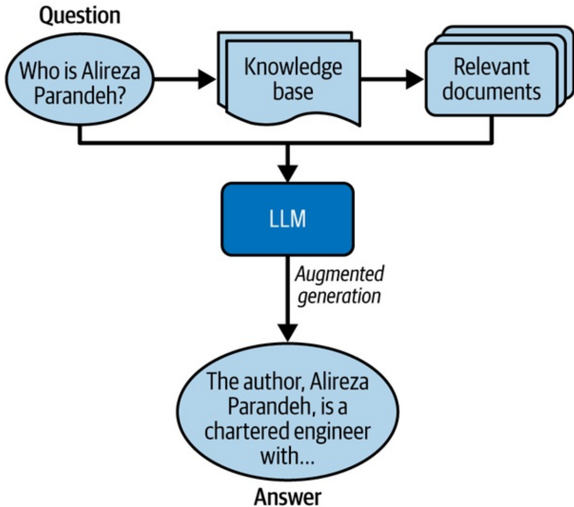
Figure 5-7. RAG
